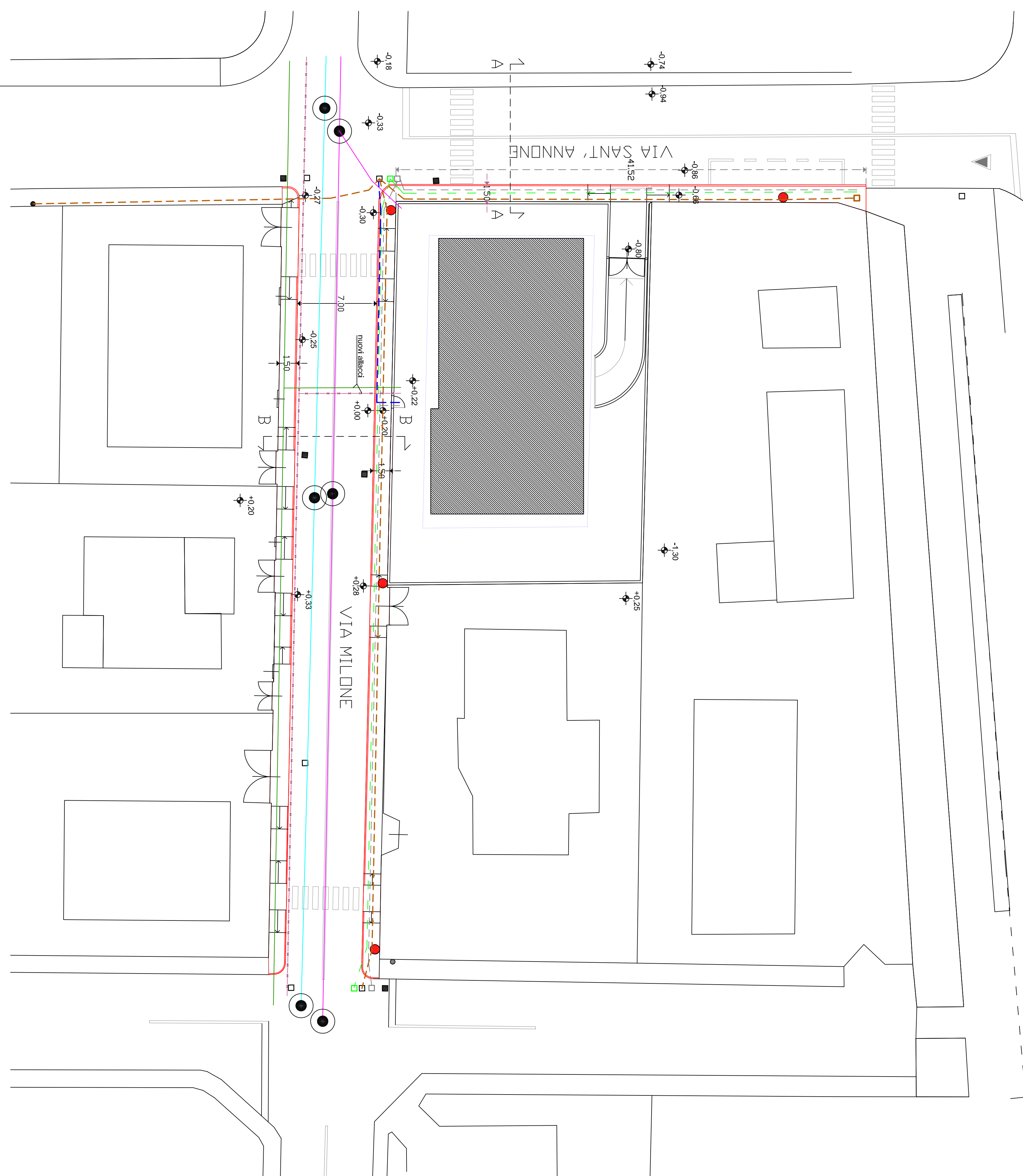
PIANTA 1 / 200
